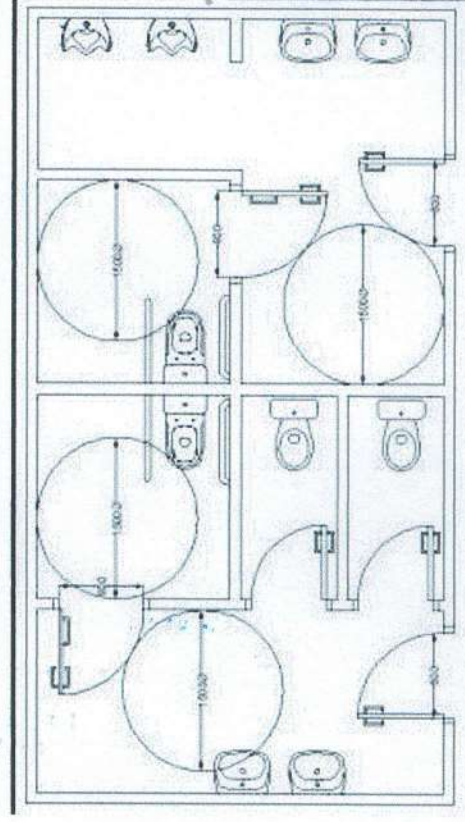
1. Виділення додаткового приміщення, препланування санвузлів
